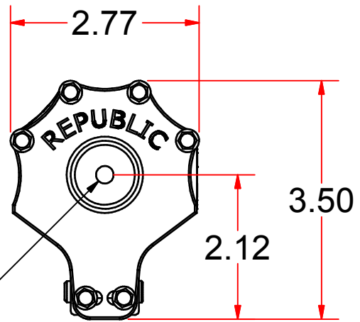
VIEW A-A
