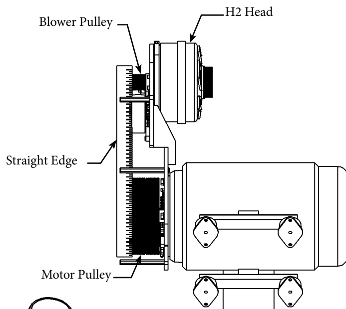
View A-A
